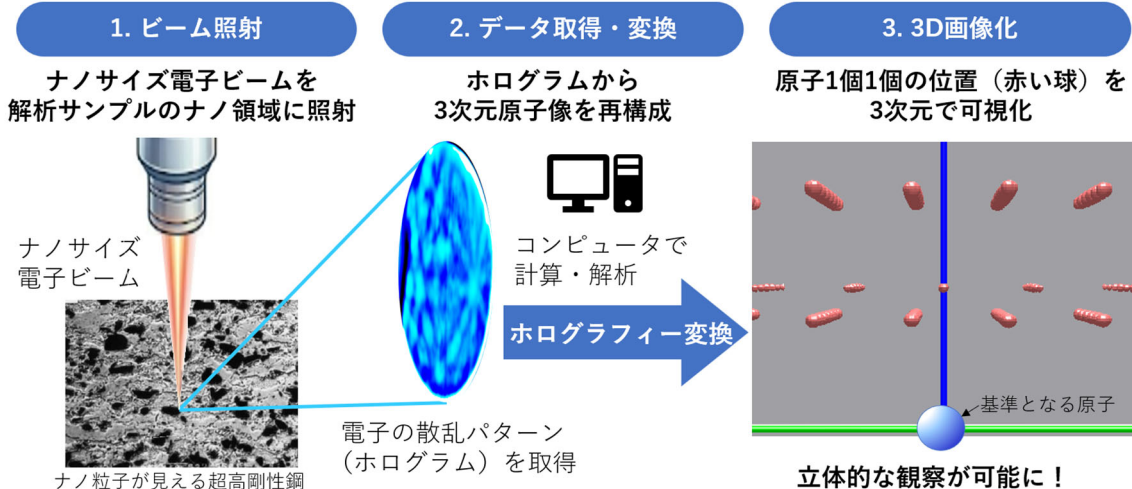
図1 原子ホログラフィー顕微鏡の概念図
