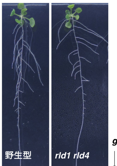
図. 通常、植物の根は重力の方向を感じ取り、重力の方向に従って伸びる重力屈性を示す（左：野生型）が、 rld1 rld4 二重変異体（右）では、重力屈性が弱く、側根が水平方向に向かう傾向が見られる。
